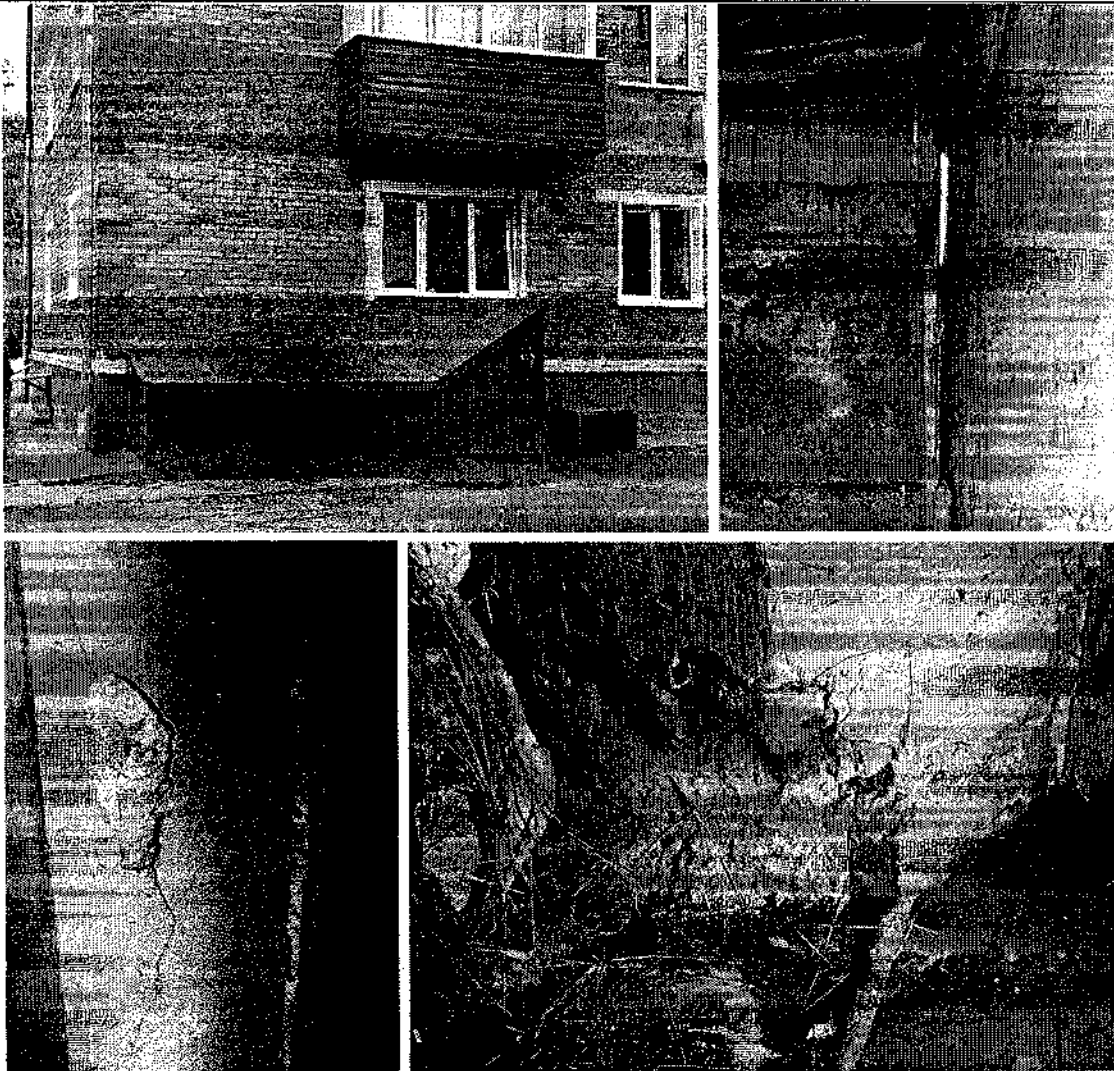
Фото 5 – 7. Локальные разрушения защитного штукатурного слоя цокольной части здания. Дефект эксплуатационного характера. Вызван промерзанием насыщенной влагой кладки и дальнейшим её разрушением, а также внешними механическими воздействиями (включая атмосферные осадки).
